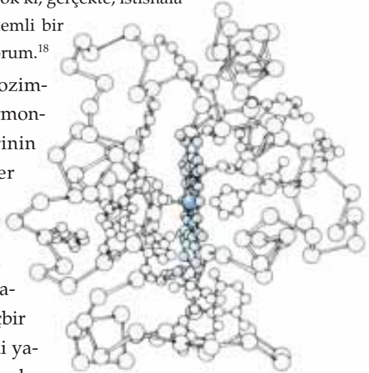
Kompleks yapısıyla Sitokrom C proteini
