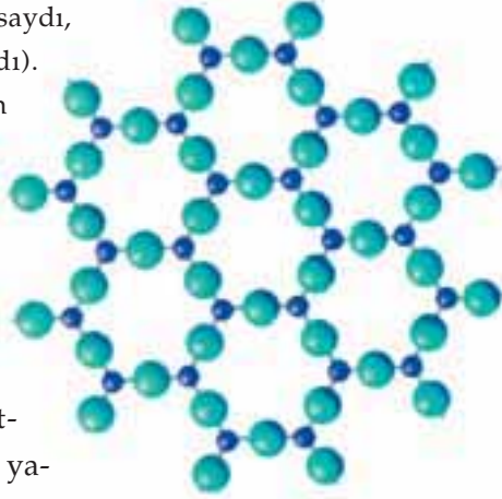
Silisyum elementinin moleküler yapısı
