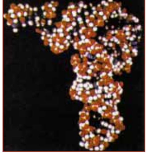
RNA sarmalı
